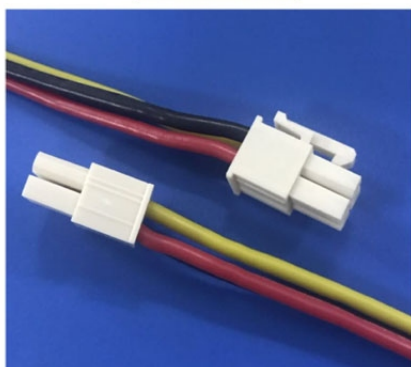
MOLEX5557-4P(2*2)
