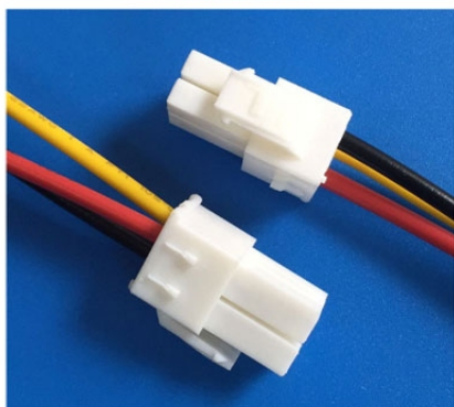
AMP177900-1
