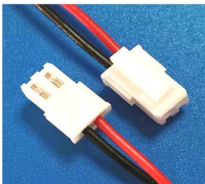
YHSMH250-2P
